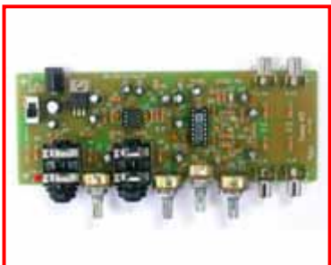
マイクエコープリアンプ
